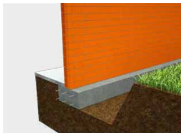
1 Fondazione in c.a. di sezione di larghezza ben superiore alla muratura
